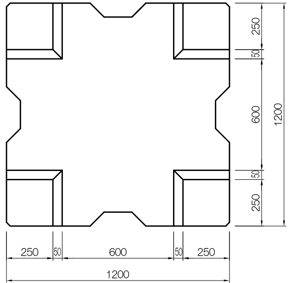
● 底面図
